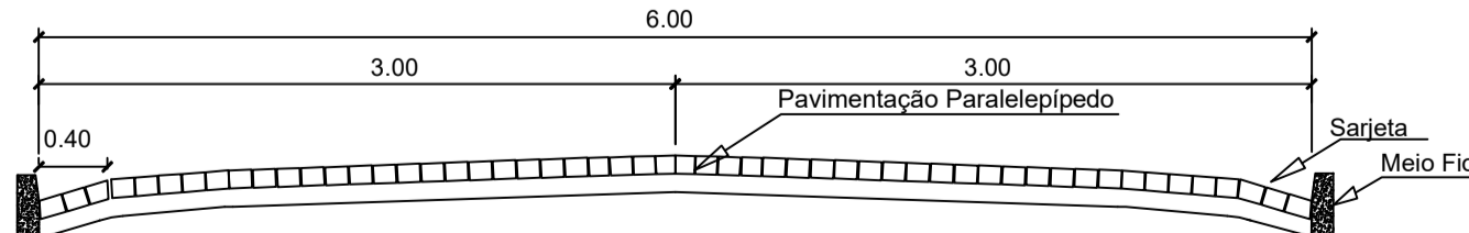
FIG. 04a - PAVIMENTAÇÃO SEÇÃO TIPO RUA PROJETADA 01
